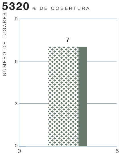
Figura 1.4 Frecuencia de cobertura del tipo de hábitat 5320 en LIC. La variable denominada porcentaje de cobertura expresa la superficie que ocupa un tipo de hábitat con respecto a la superficie total de un determinado LIC..
